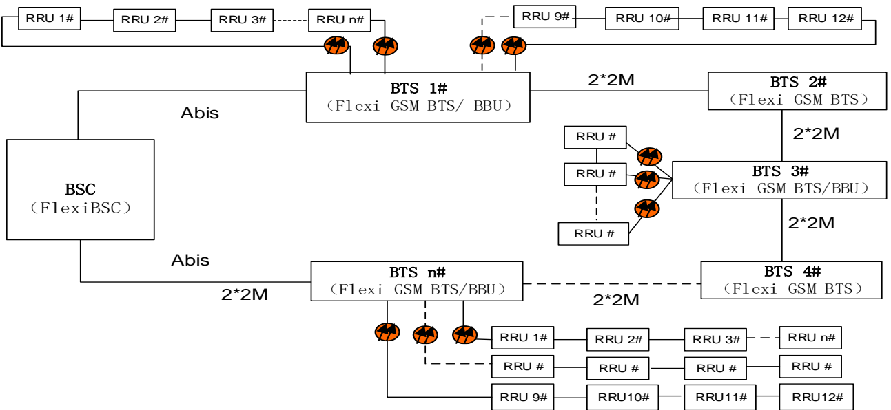
图1：BTS与传输端口连接图
